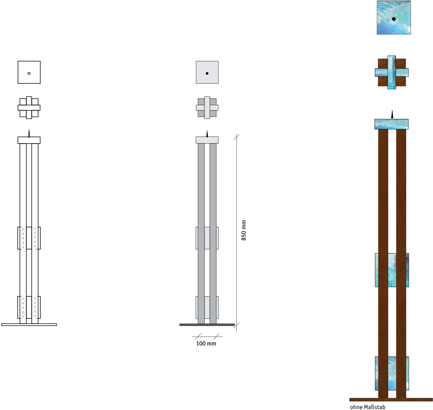
Kerzenständer (optional) M 1:10
